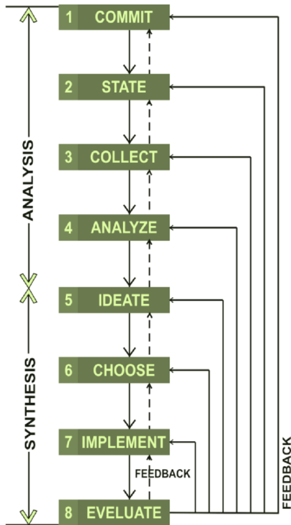
Gambar 1. Bagan Metodologi Desain
