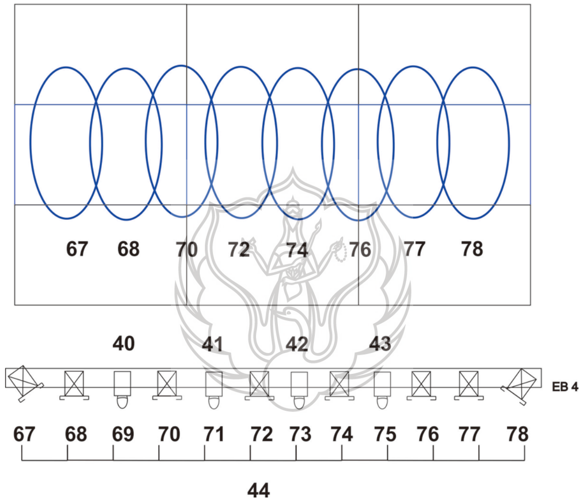
Gambar 7. Sketsa Floor Plan Batten 4 (Sketsa : Krisna Megumi dan Alfian Dion, 2018)
