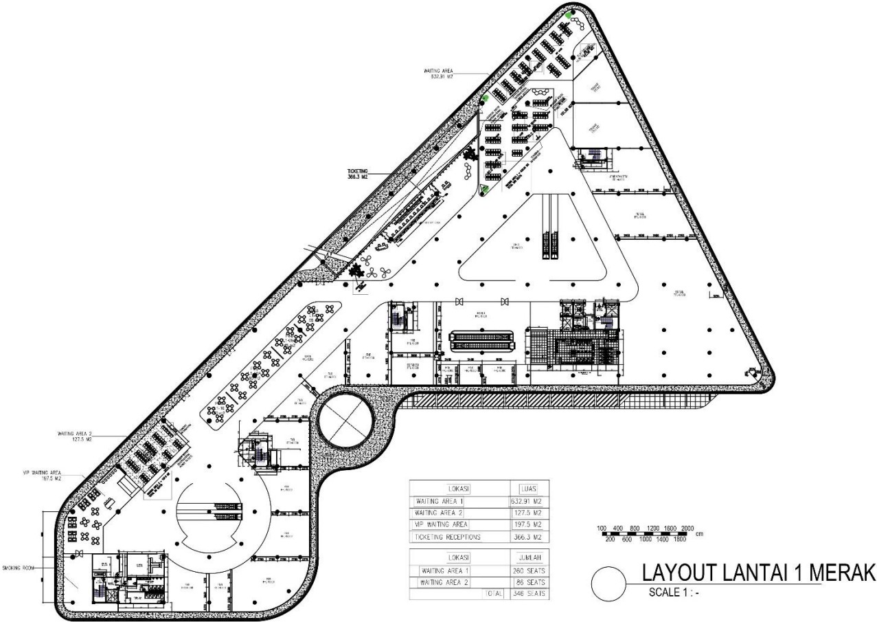
Layout Lantai 1 Pelabuhan Eksekutif Merak
